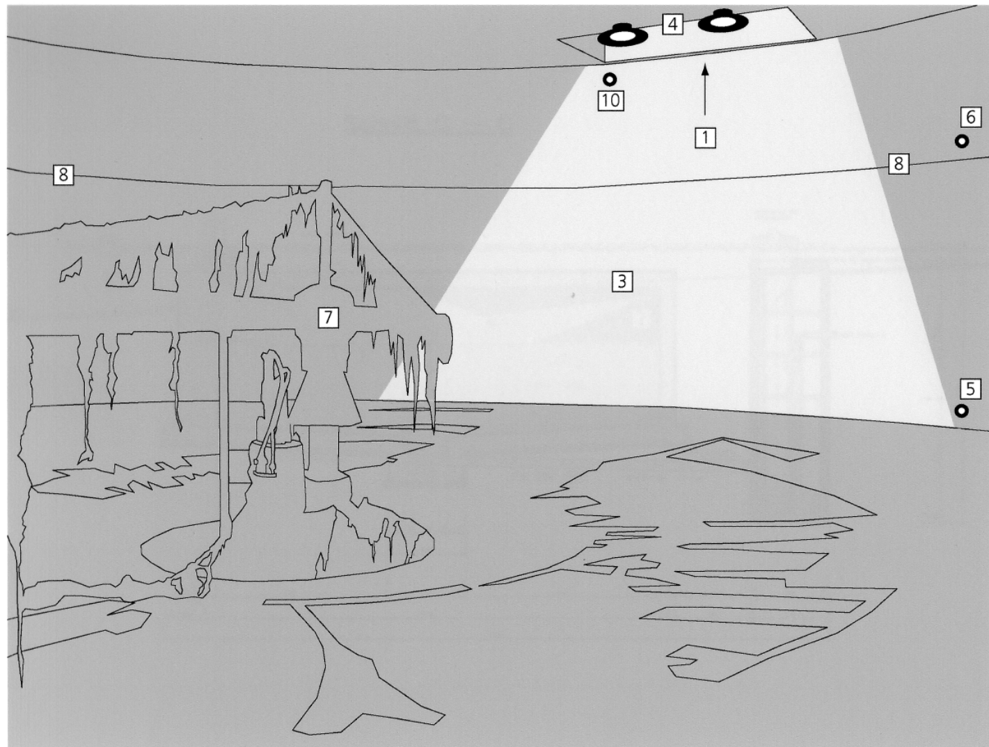
Regenbecken – Innenansicht
